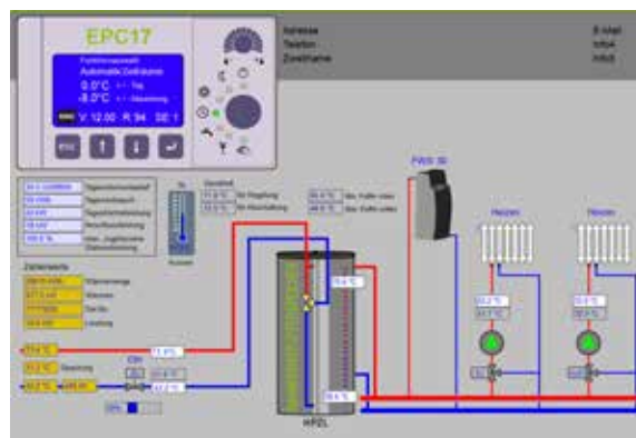
Abb. 39: Bildschirmanzeige Abnehmer
